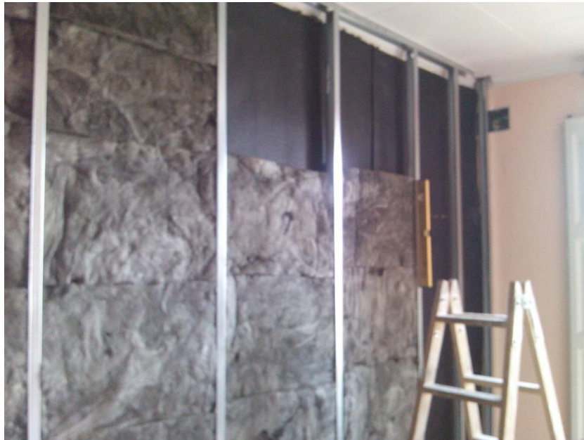
Primena zvučne izolacije AIT PR 3.5 u sistemima zidnih obloga
