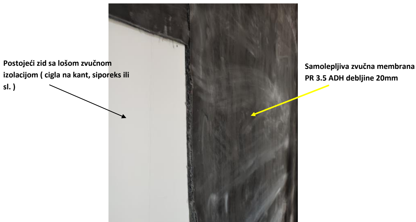
Popravka zvučne izolacije postojećeg zida samolepljivom membranom AIT PR 3.5
